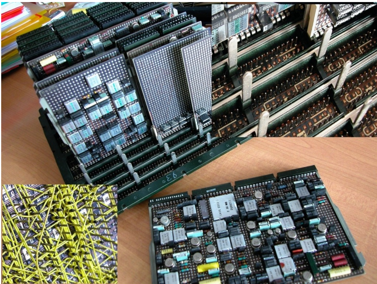
Hier Backplane und Steckkarten einer IBM370 (Bild: Wikipedia)
